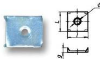
755-06 Ø=3 L=17 l=15 g=3,5 755-12 Ø=3,5 L=13 l=13 g=3
